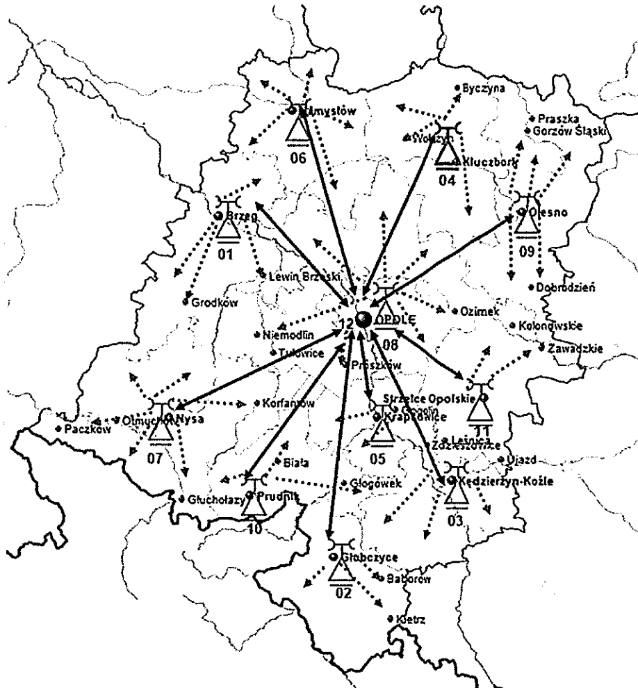
§ 9. Tabela kodów obszarów objętych działaniem systemu DSP-50/OC wersja Opole.
